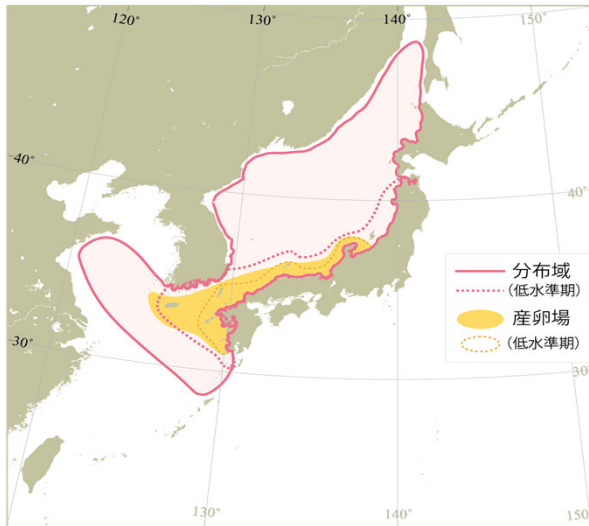
図1 分布域
