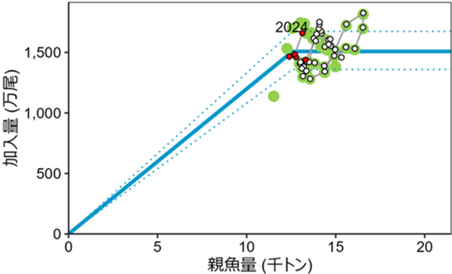
図6 再生産関係
