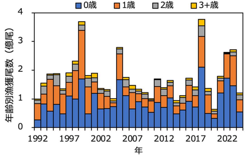
図3 年齢別漁獲尾数の推移
