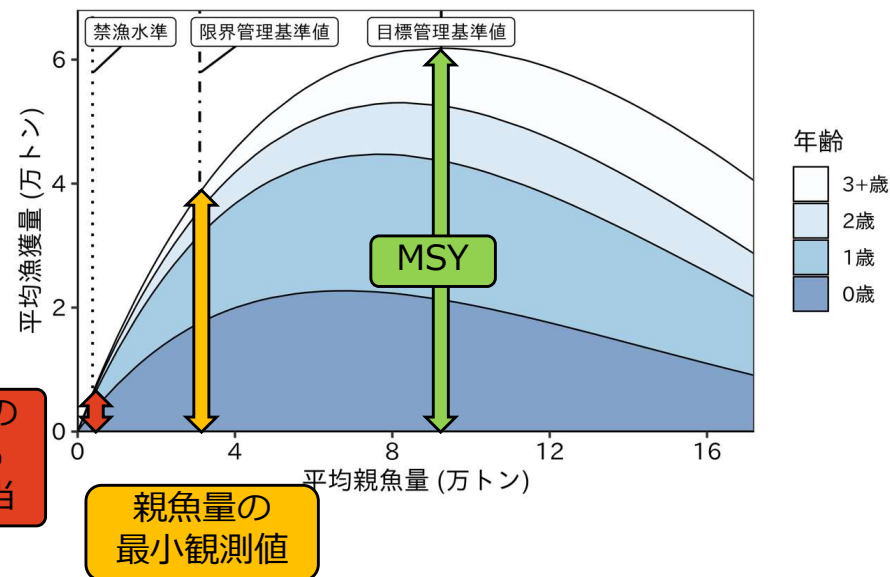
図9 管理基準値と禁漁水準
