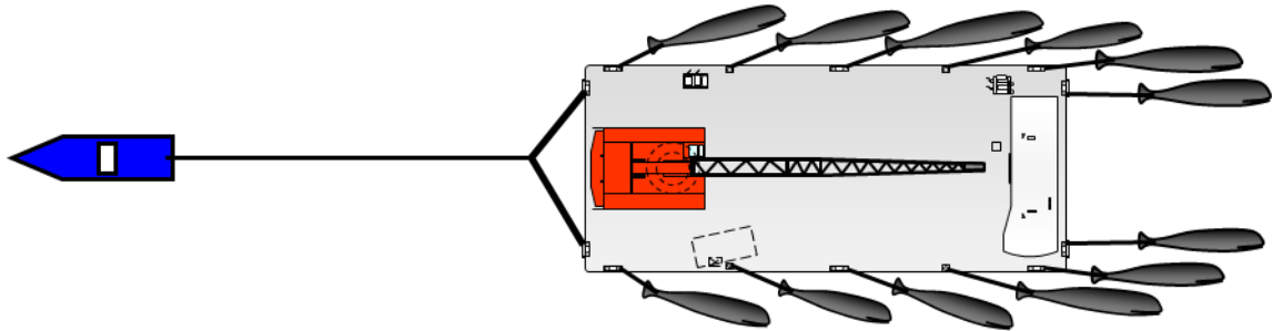
図V-4 鯨体の台船への係留
