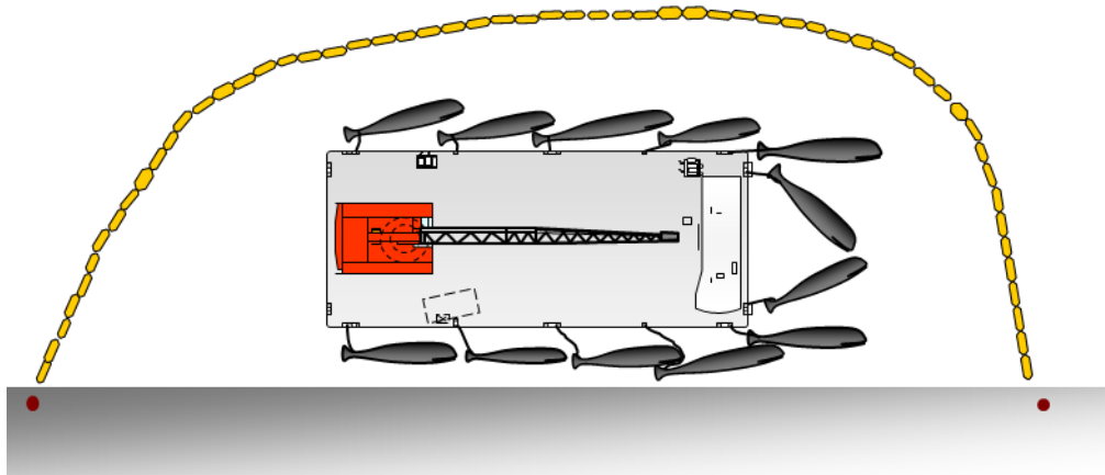
図V-13 オイルフェンスの設置
