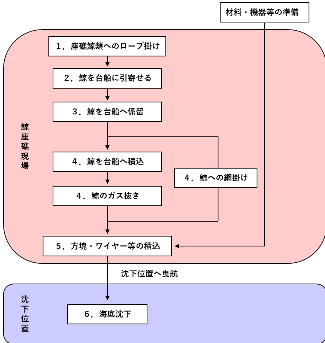
図 V-1 海底沈下作業フロー（通常対応）
