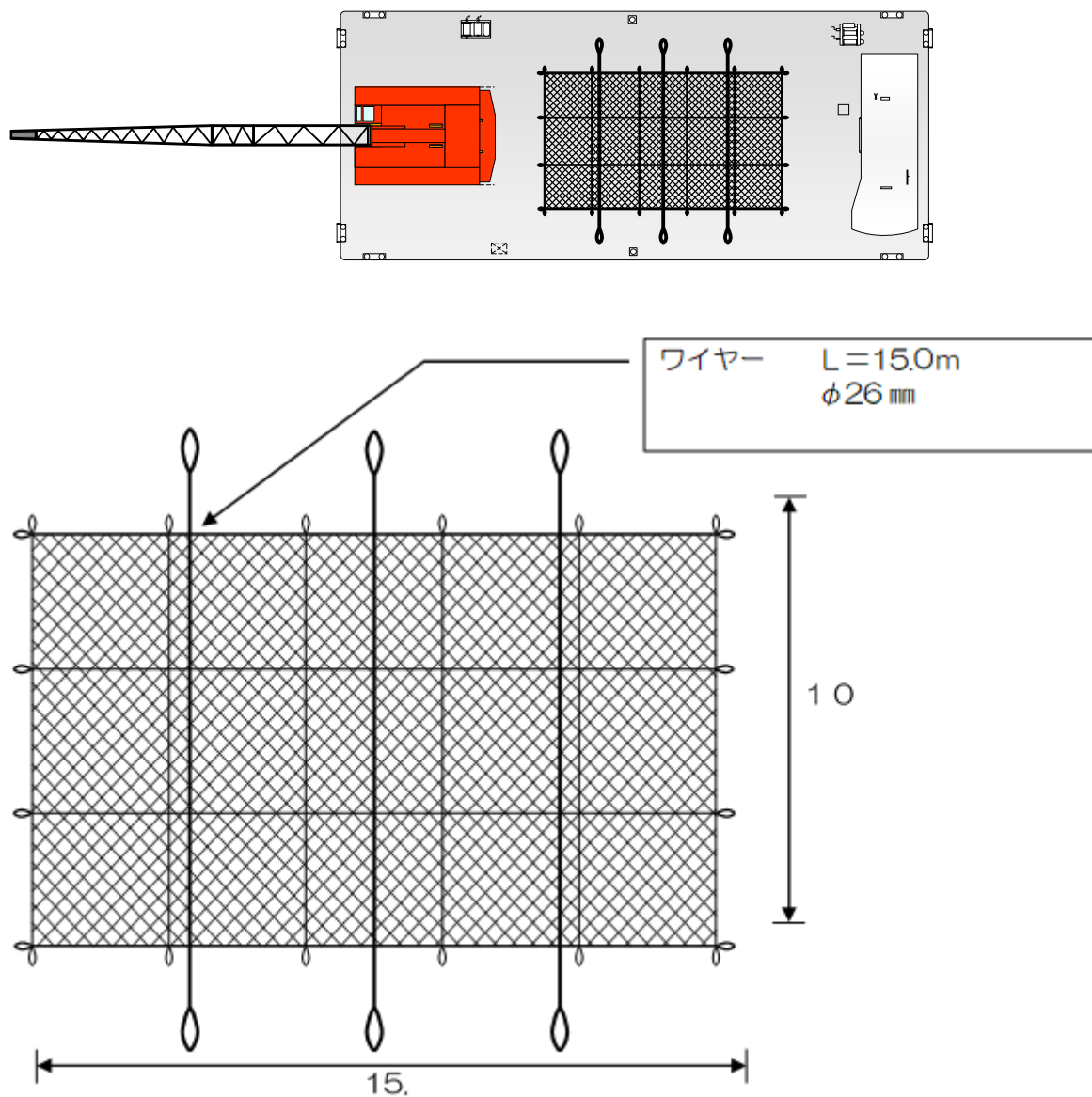
図V-5 台船上にワイヤー及び漁網を敷設
